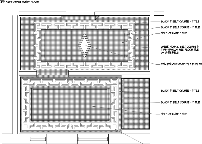
12 TILE PATTERN A4 SCALE: 1/2" = 1'-0"
